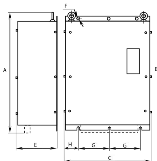
Рисунок 2 93...160 кВт (125...200H) IP54
