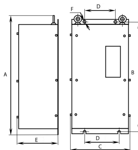
Рисунок 2 37...75 кВт (050...100H) IP20 37...93 кВт (050...125K) IP20
