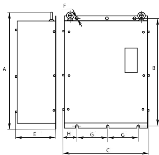
Рисунок 3 93...160 кВт(125...200H) IP20 110...160 кВт(150...200K) IP20
