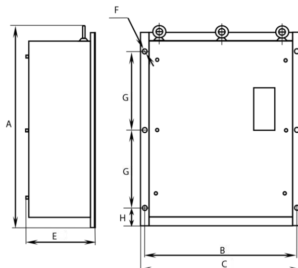
Рисунок 4 185...500 кВт (250...600H) IP20 185...500 кВт (250...600K) IP20
