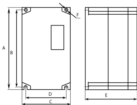
Рисунок 1 0,75...30 кВт (001...040H) IP20
